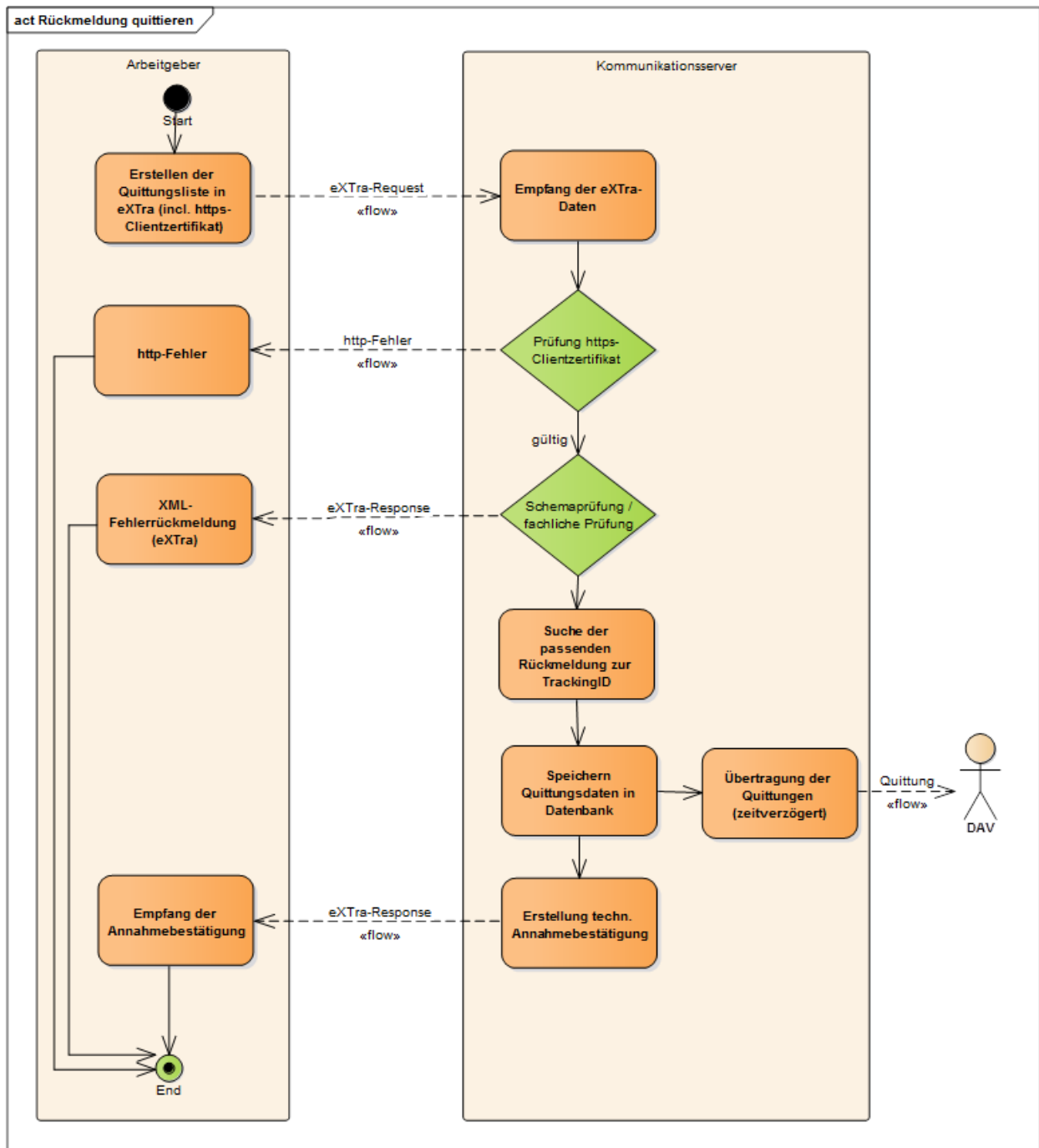
Abbildung 6: Flussdiagramm zum Verarbeitungsablauf der Empfangsquittungen
